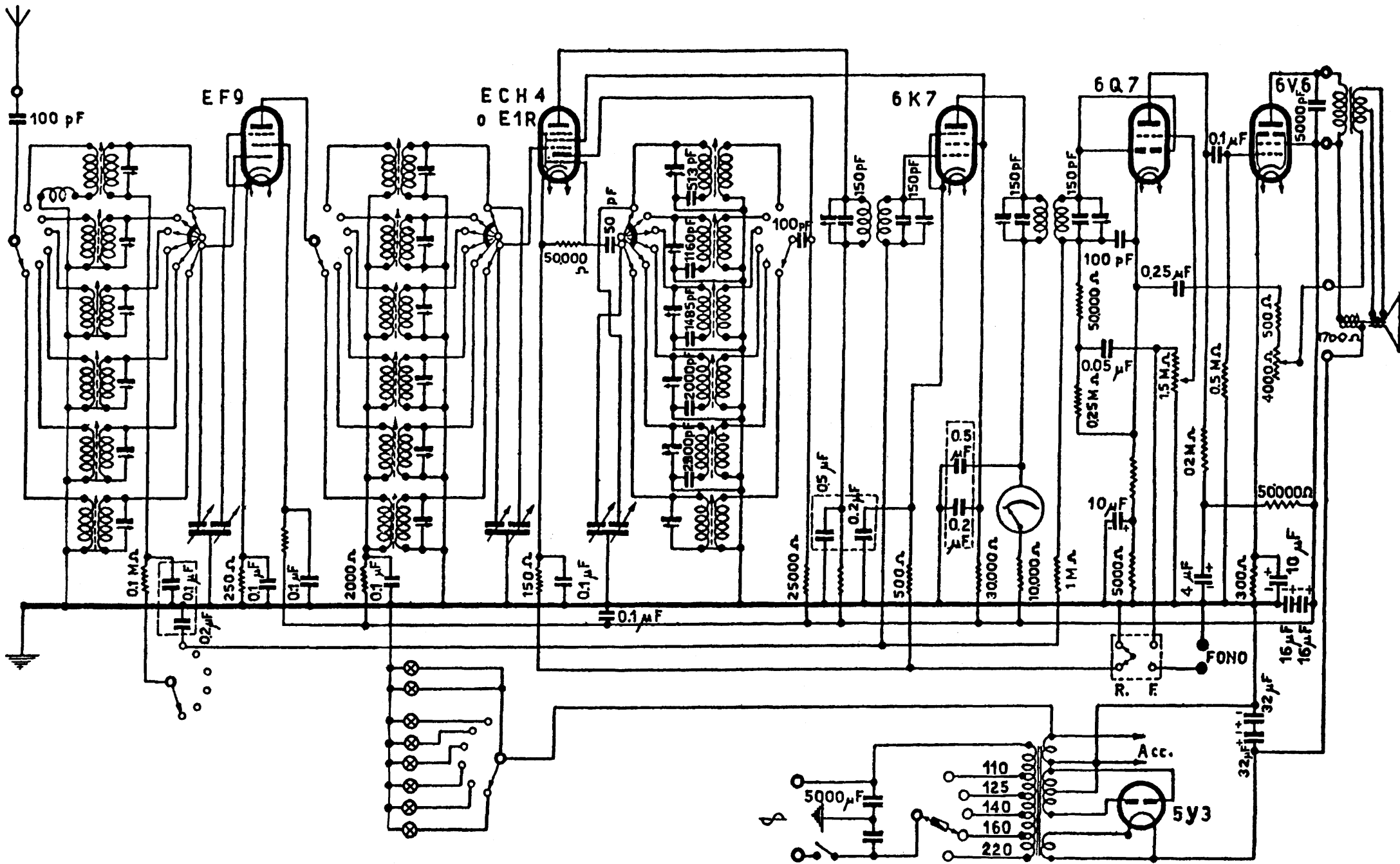
4 - ALLOCCHIO, BACCHINI e C. - MOD. 615. Gamme di ricezione: da 190 a 570 m, da 12 a 19 m, da 17 a 26 m, da 23 a 36 m, da 32 a 50 m e da 49 a 70 m. Sensibilità da 5 a 10 microvolt. Potenza: 4,2 W. MF: 465 kc/s. Produzione 1946.
